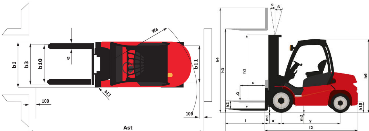
MI 30 G ST5 - Rysunek wymiarowy
